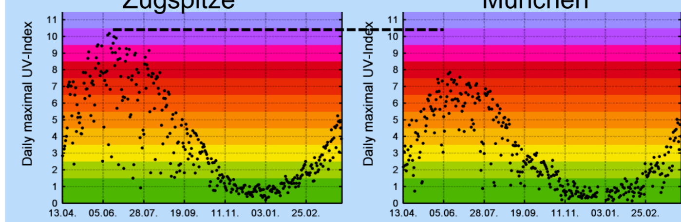
UV – Index April 2017 – April 2018 Zugspitze München
